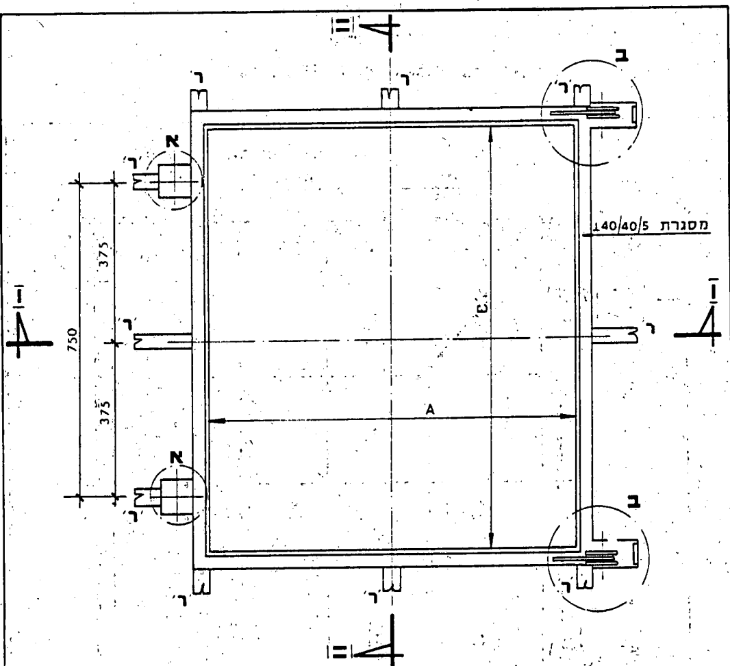
תנוחת המסגרת
