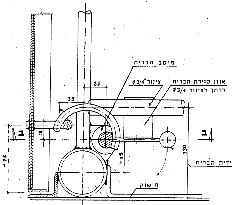
פרט מנגנון הנועילה
