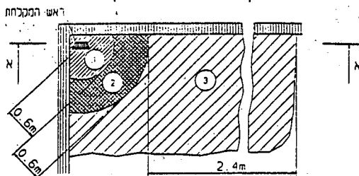
חתך א-א
